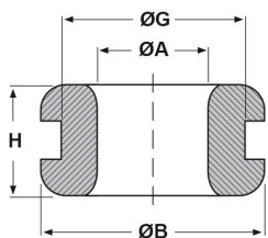
foro svasato
