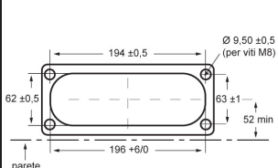
DIMA FORI PARETE
