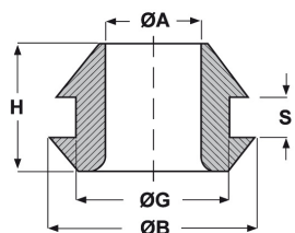
DKA 8/11,5/15-1,5
