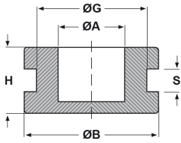
forma piana
